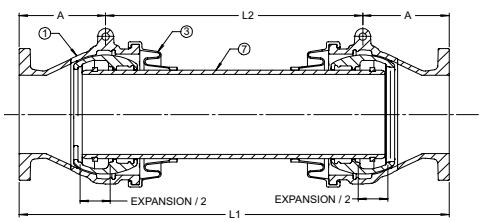
SECTION A-A FLANGE X FLANGE
